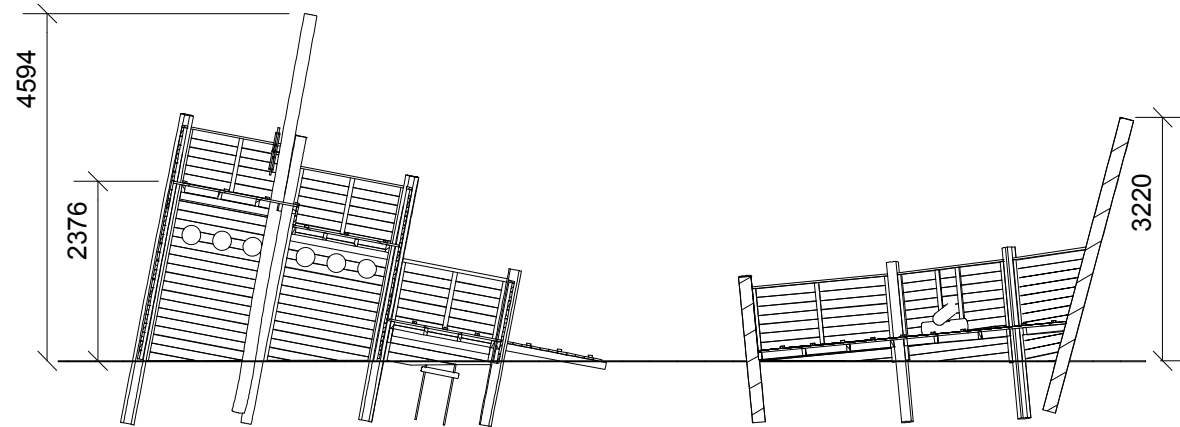
A-A ( 1 : 100 )
